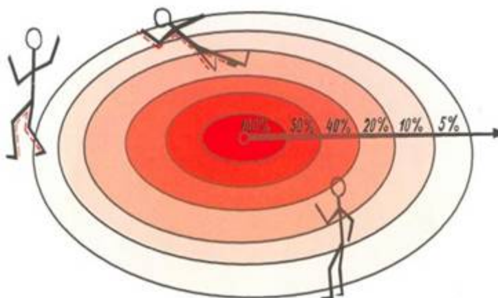
Рис.10 Опасная зона шаговых напряжений
